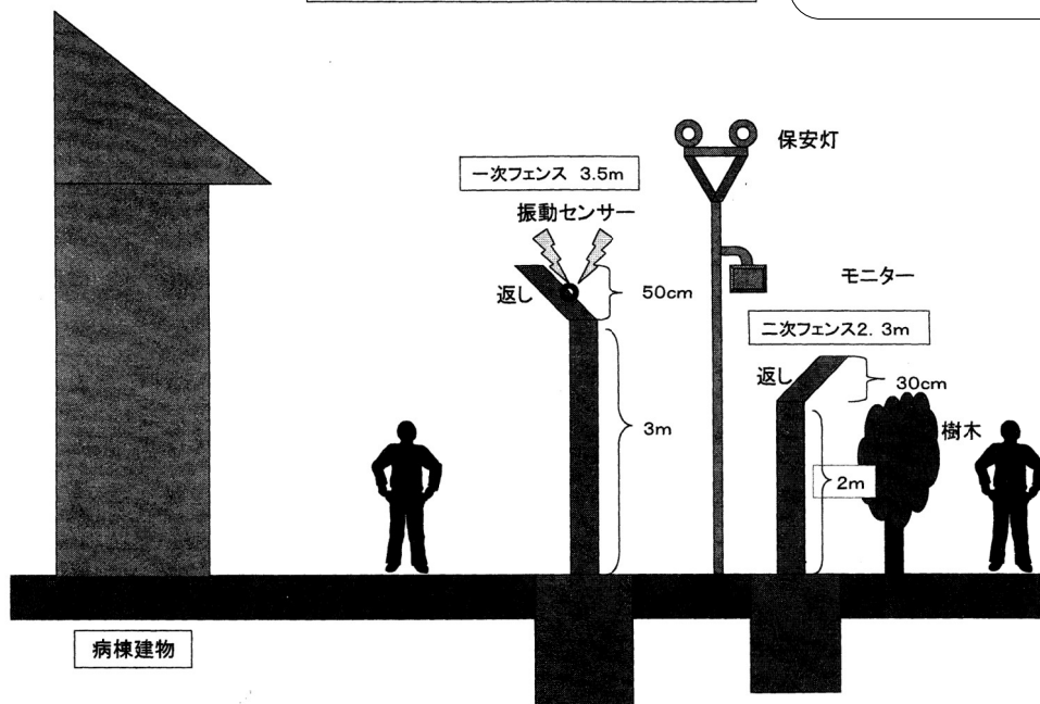
フェンス及びセンサー等の設置図
